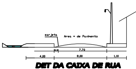
CORTE A-A (TRANSVERSAL) PAVIMENTO TIPO S/ ESCALA
