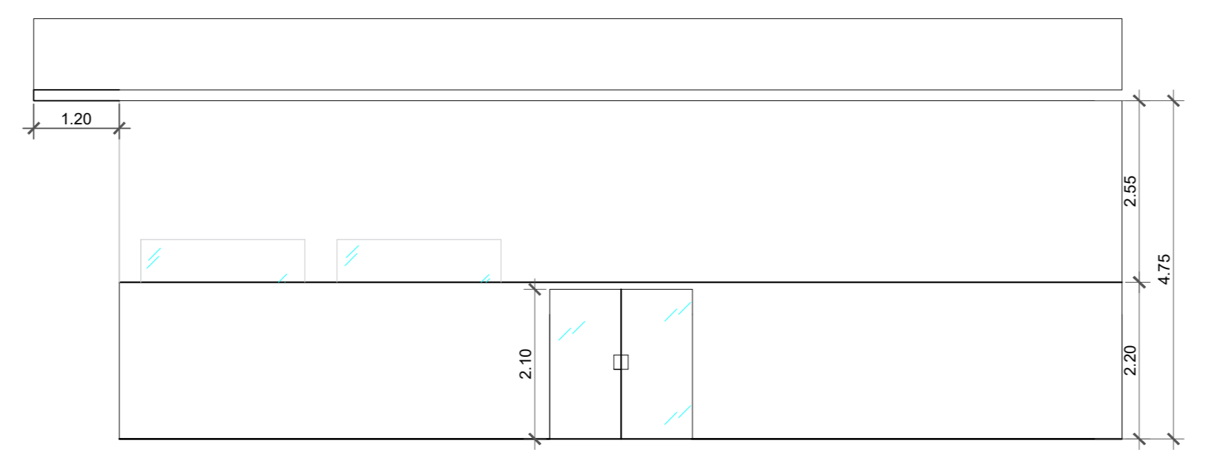
FACHADA D Esc.:1/75
