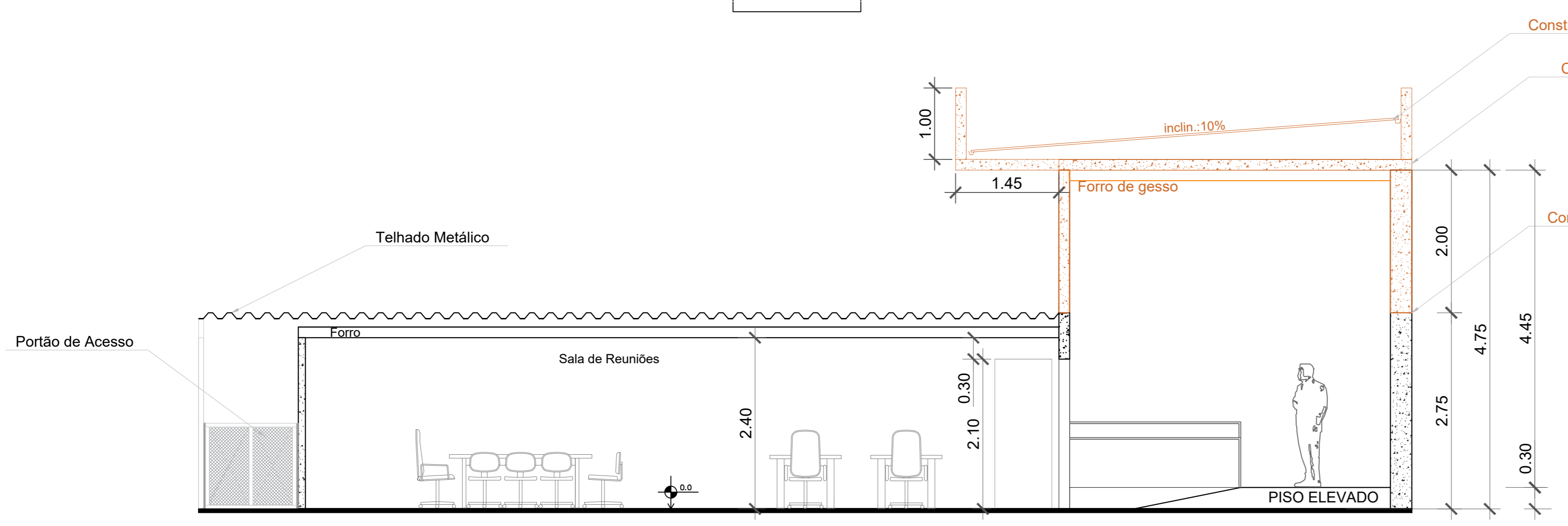
Corte 1 Esc.1/50
