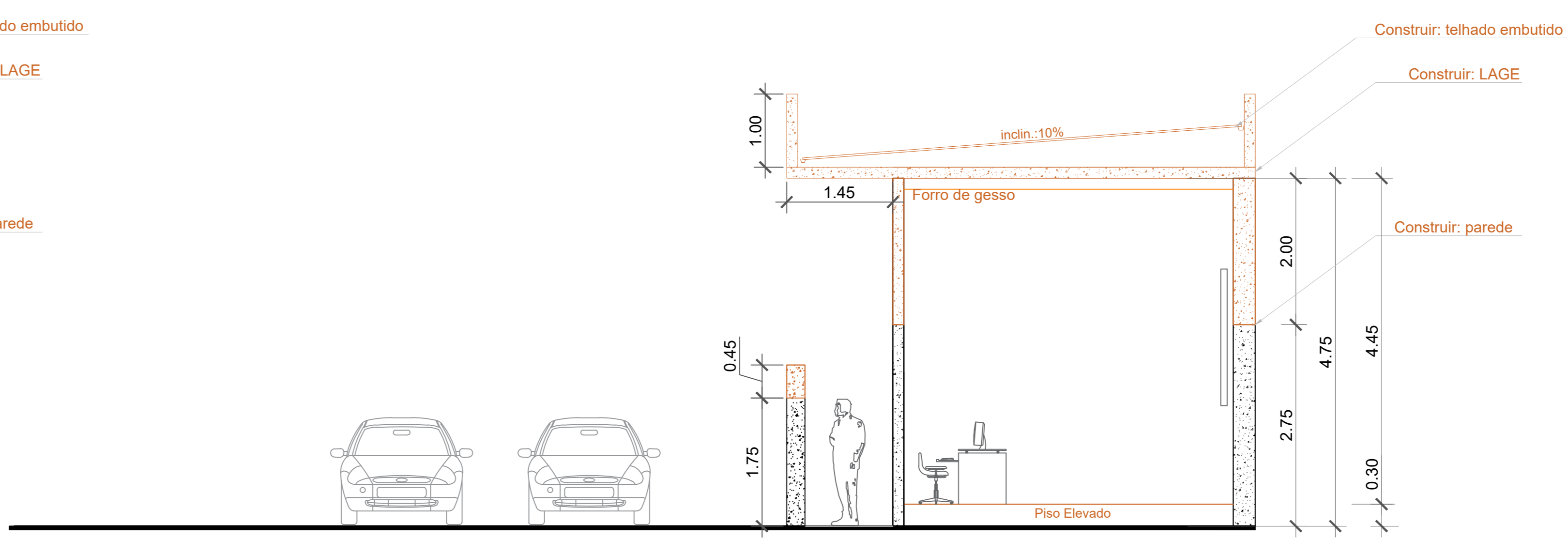
Corte 2 Esc.1/50
