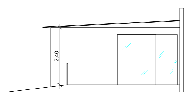
FACHADA B Esc.:1/75
