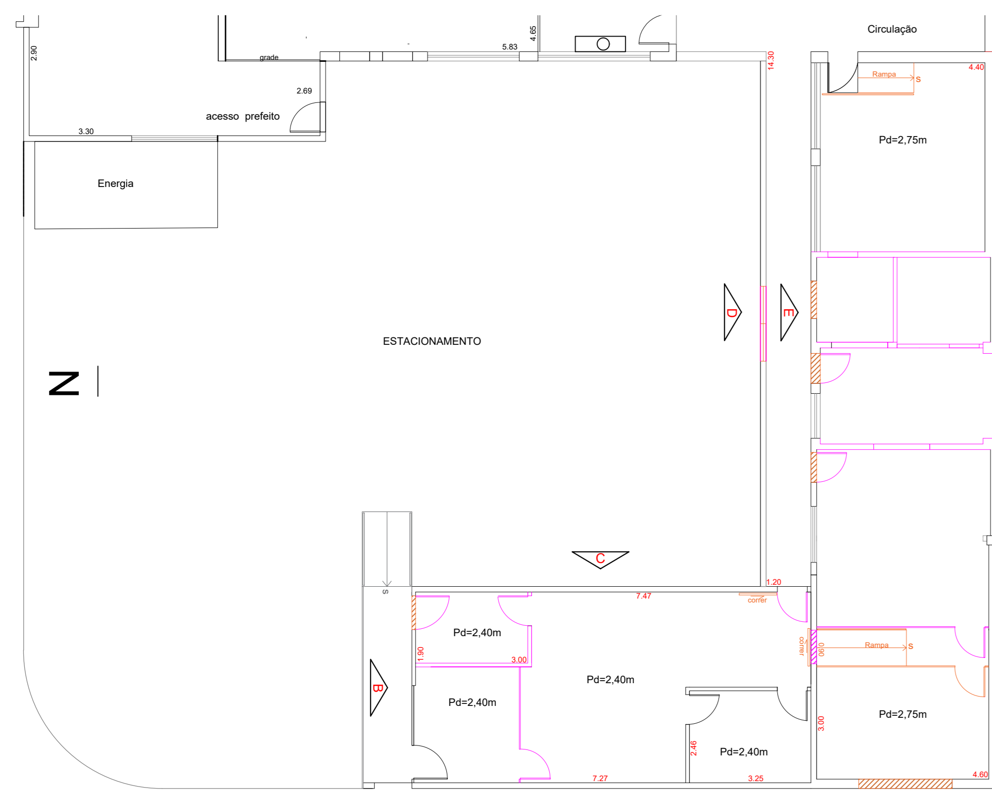
DEMOLIR/CONSTRUIR Esc.1/100
