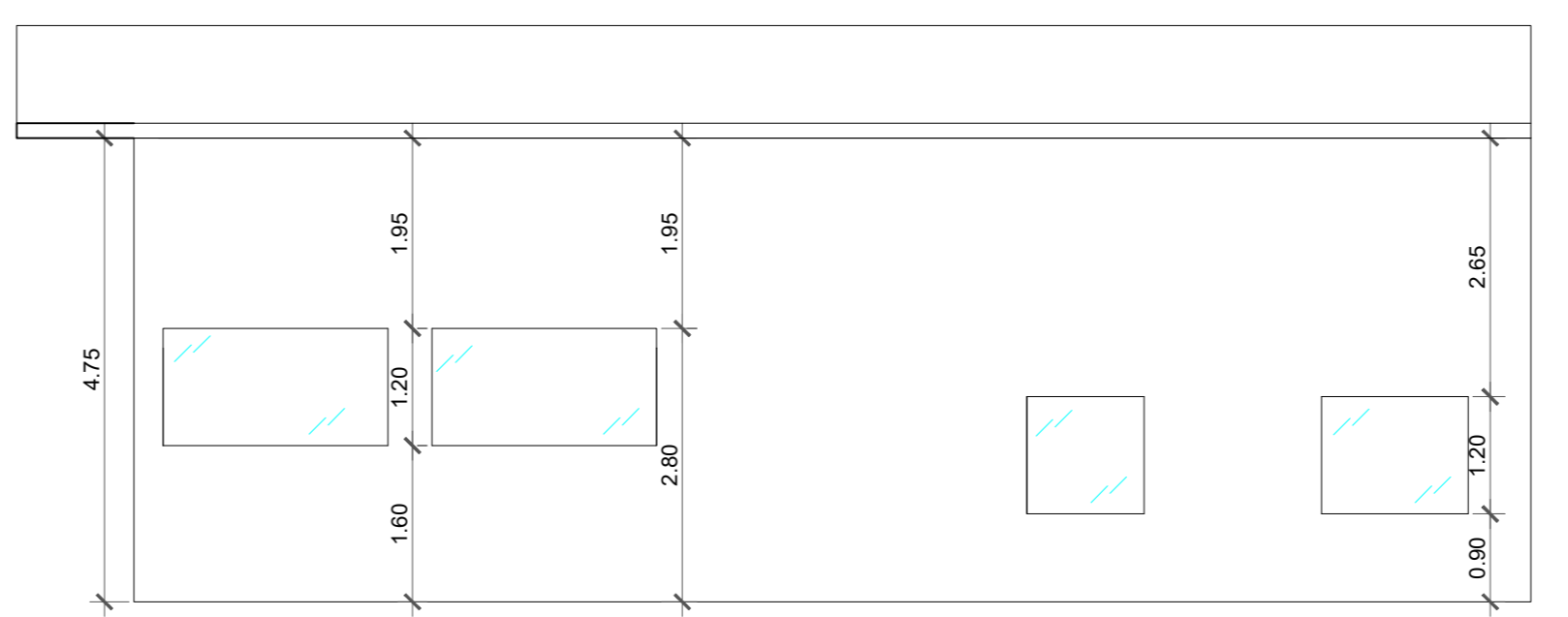
FACHADA E Esc.:1/75
