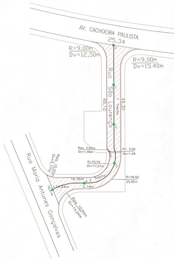
DET DA CX DE RUA - 1º TRECHO
