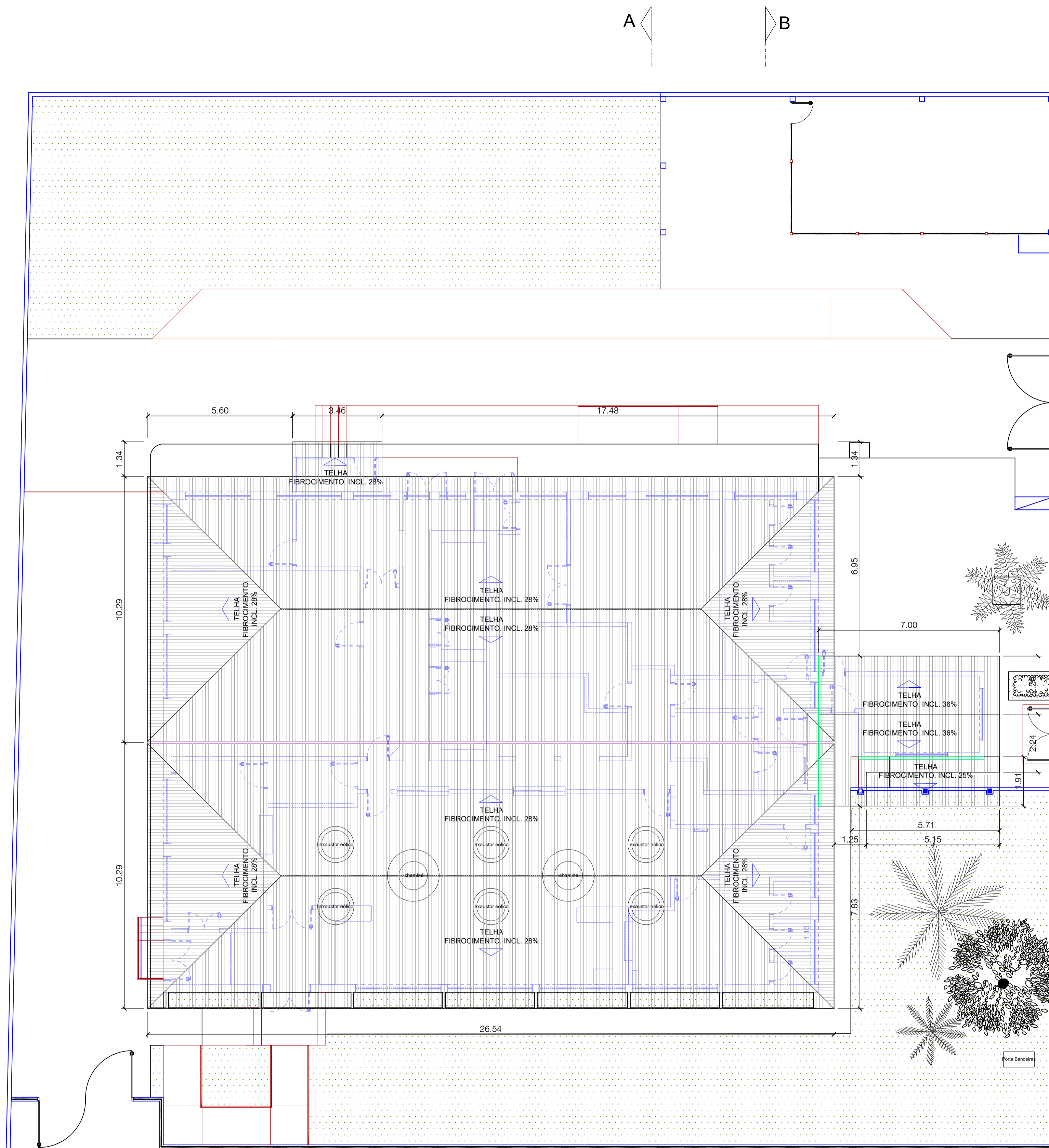
PLANTA COBERTURA ESCALA 1:00
