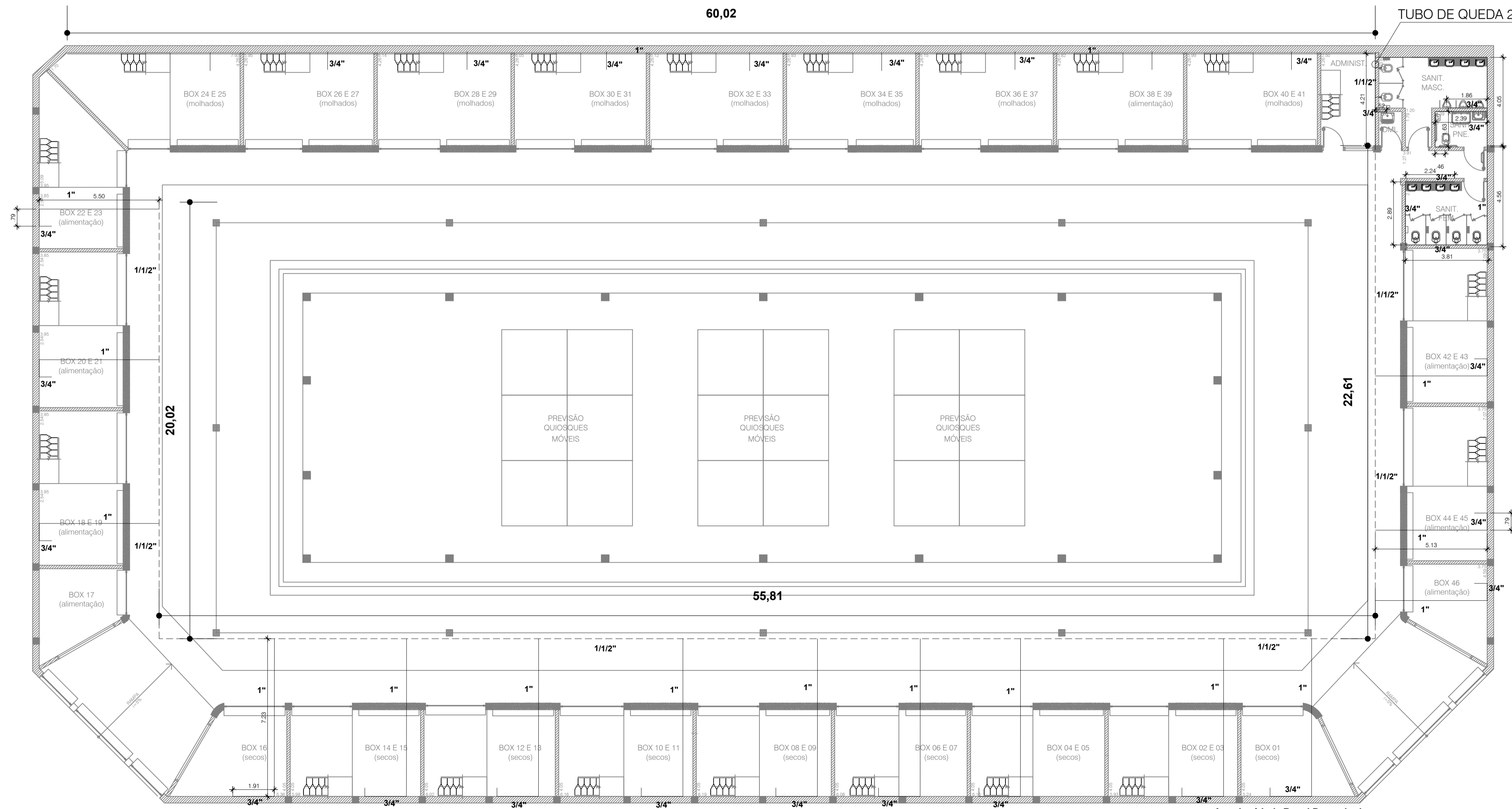
PLANTA-PROJETO HIDRÁULICA ESCALA 1:125
