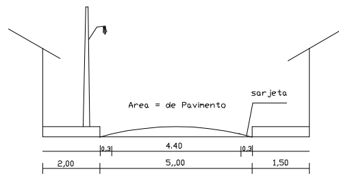
DET DA CAIXA DE RUA
