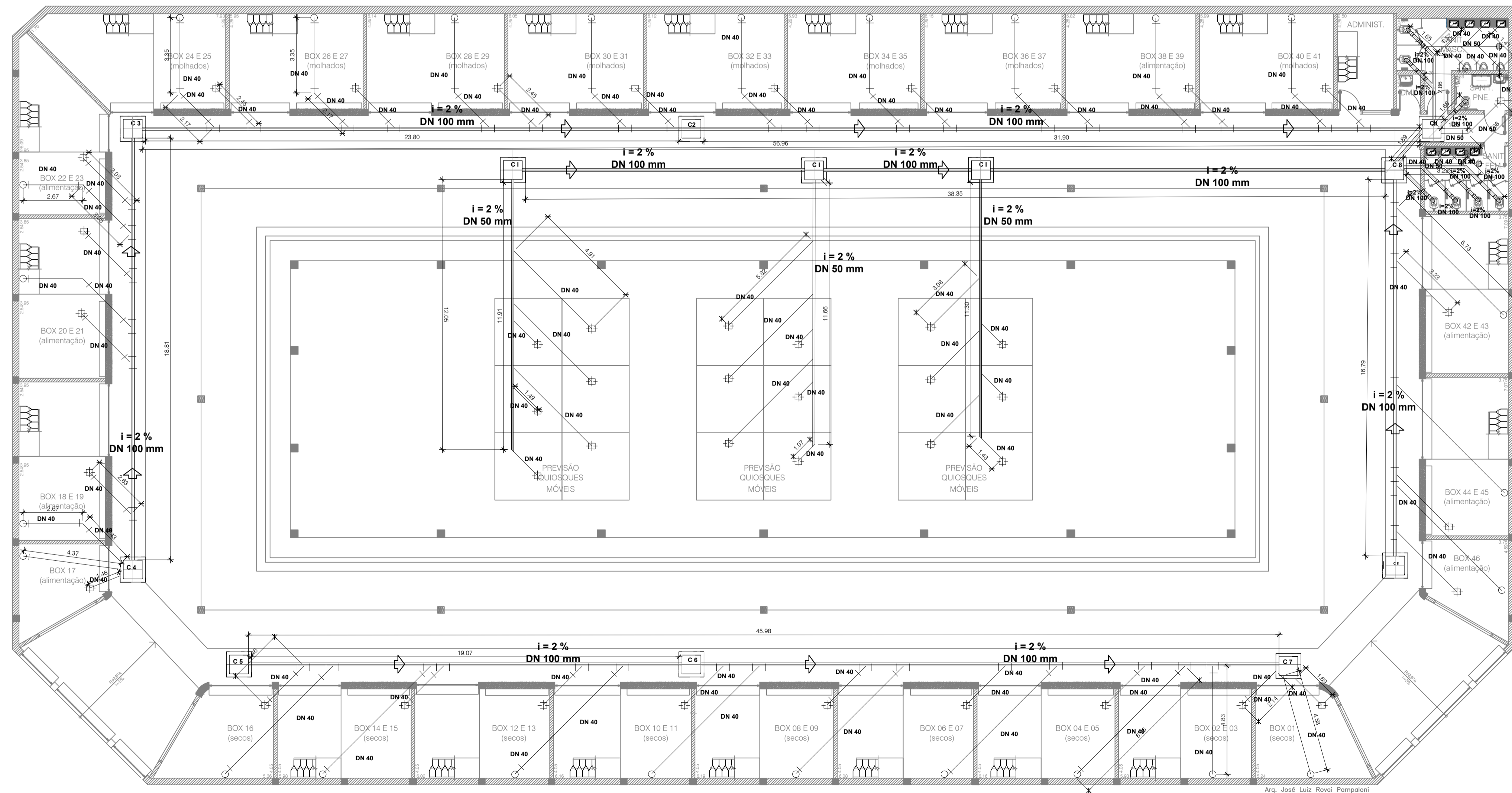
PLANTA - PROPOSTA DE ESGOTO ESCALA 1:125
