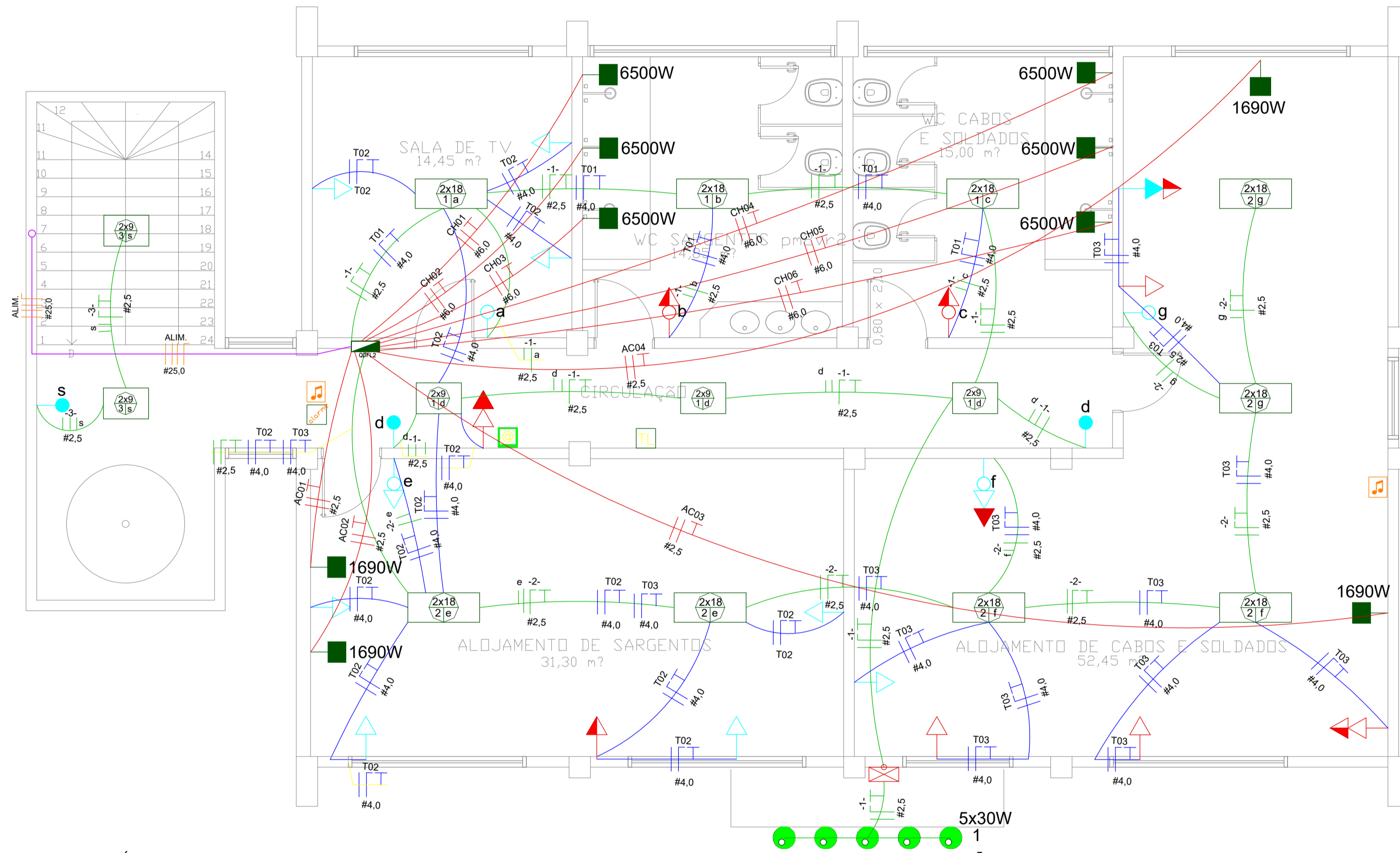
PLANTA ELÉTRICA - PAV. SUPERIOR ESCALA 1:50
