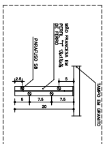
DETALHE MÃO FRANCESA ESCALA 1:5
