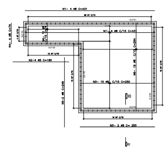
ARMAÇÃO DA FUNDAÇÃO (RADIER) - BASE DO GERADOR
