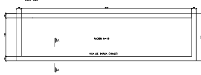
FORMA DA FUNDAÇÃO - LIXEIRA
