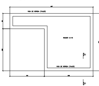
FORMA DA FUNDAÇÃO - BASE DO GERADOR
