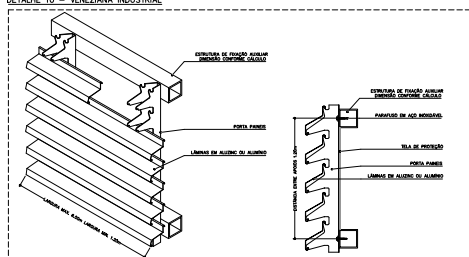
CORTE ESCALA 5/8"
