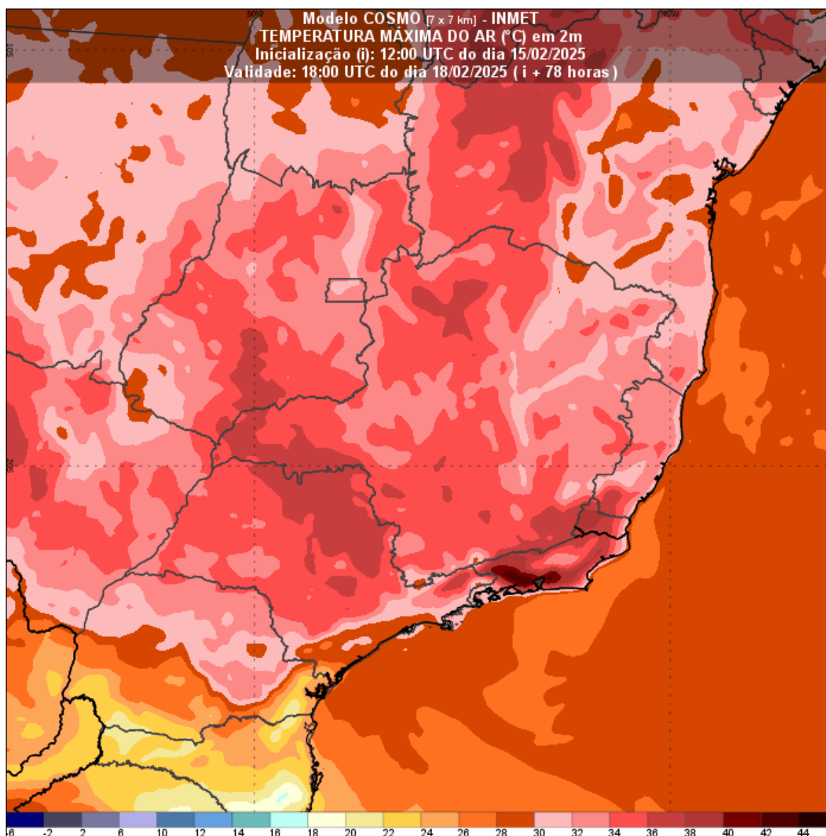
Figura 1 – Simulação do modelo COSMO/INMET para a temperatura máxima dos próximos dias.
