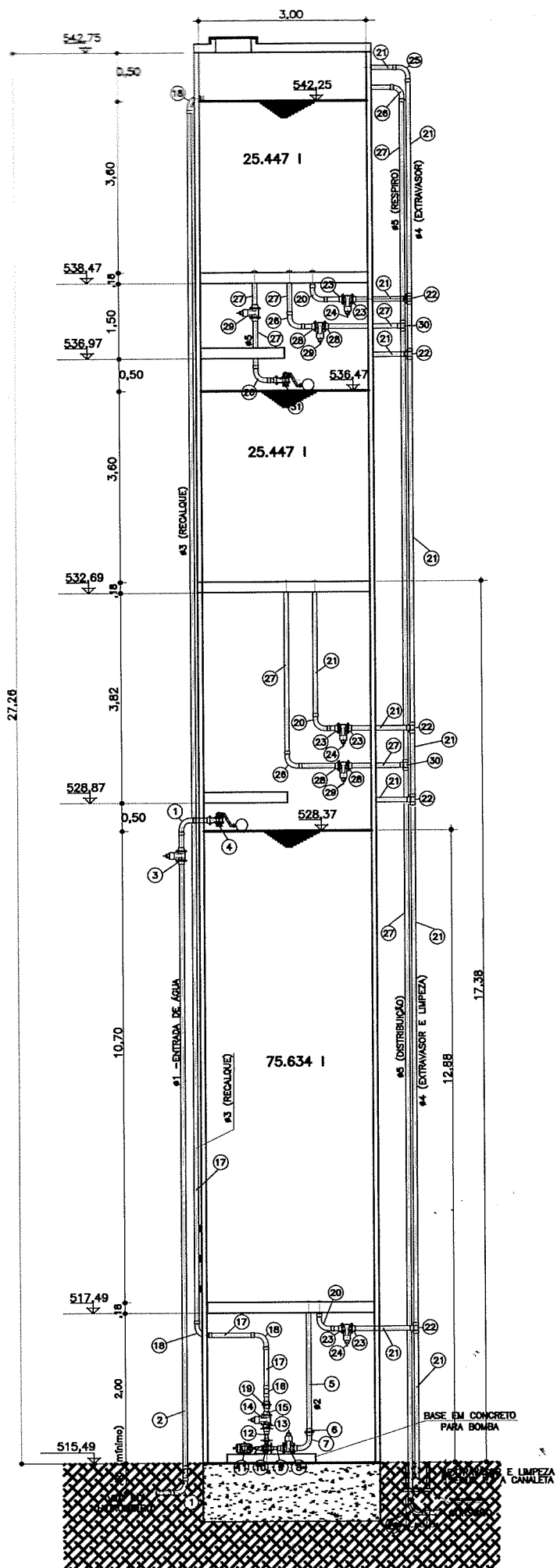
CORTE RESERVATÓRIO TIPO TORRE SEM ESCALA
